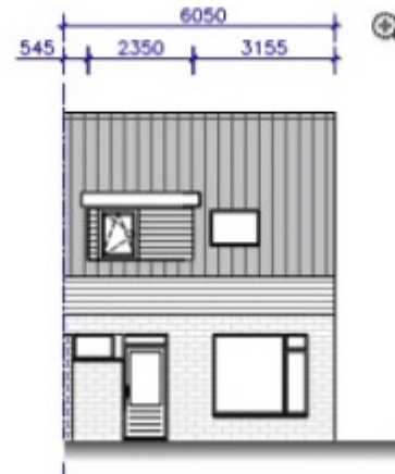
VOORGEVEL NIEUW
