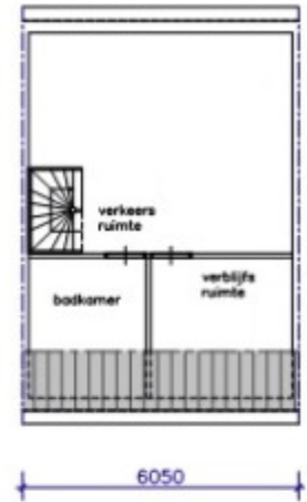
INDELING BESTAAND
