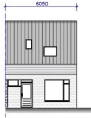
VOORGEVEL BESTAAND
