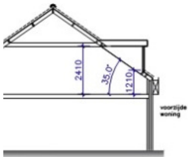
DOORSNEDE NIEUW
