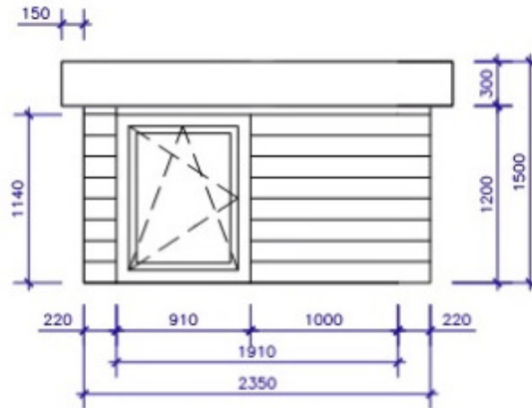
AANZICHT DAKKAPEL VOORGEVEL
