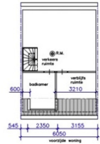
INDELING NIEUW
