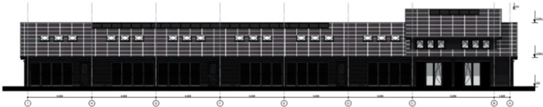
GEVELAANZICHT - Achtergevel
