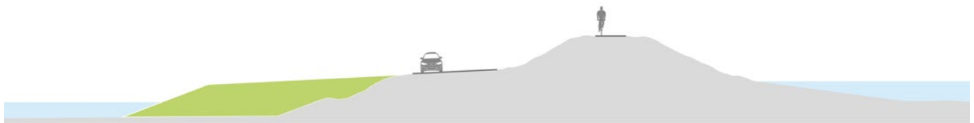
Binnenwaarts versterken ter hoogte van de braken
